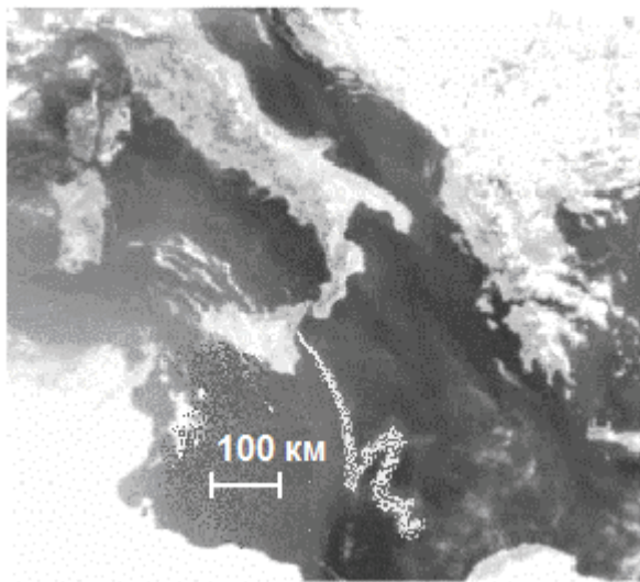
Рис. 2 Снимок из космоса 25 июля 2001 г. Шлейф газа от вулкана Этна тянется в юго-восточном направлении.
